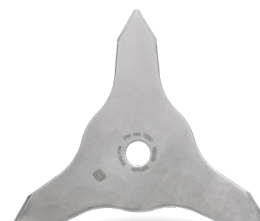
5784444-01 Disk me 3 tehe 350 x 24.5 mm
